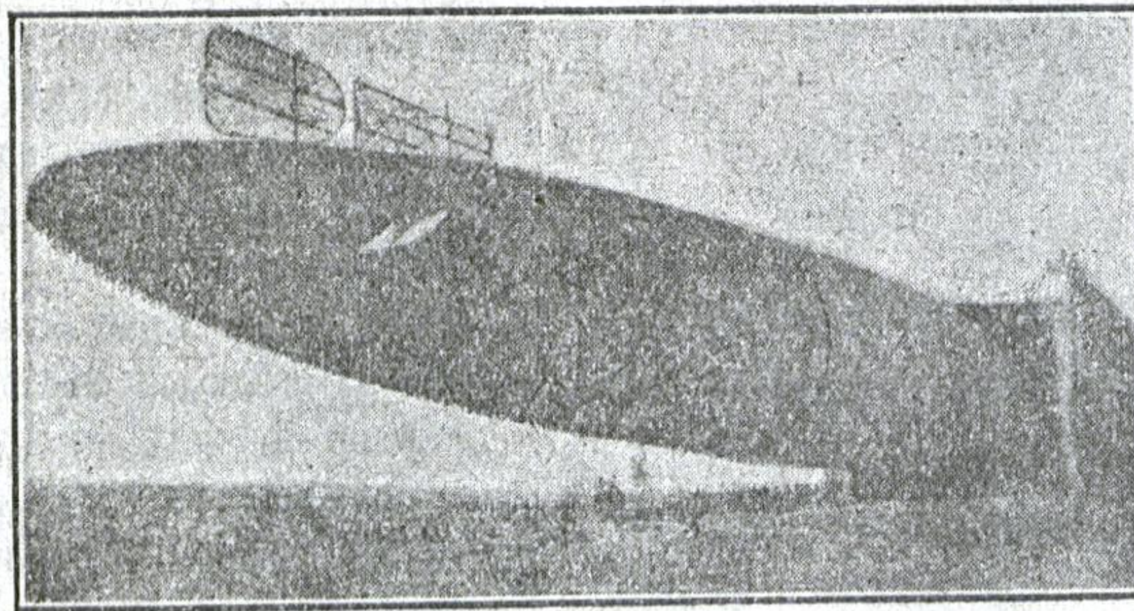
Дирижабль «Сименс—Шюттс—Ленц», с деревянным остовом, вылетает из ангара.
